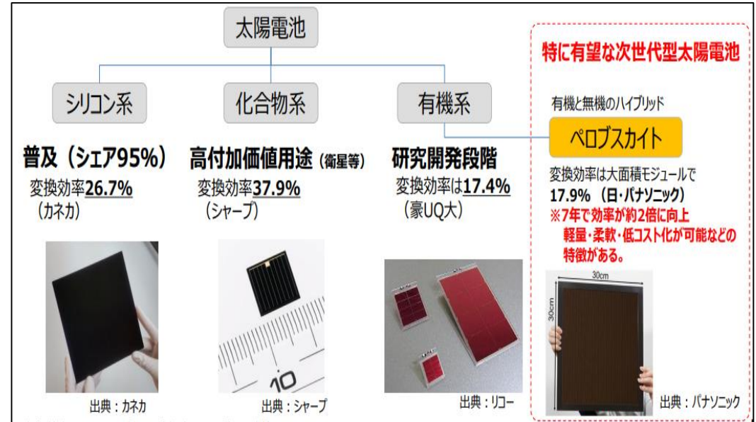
【太陽電池の種類と比較表】
