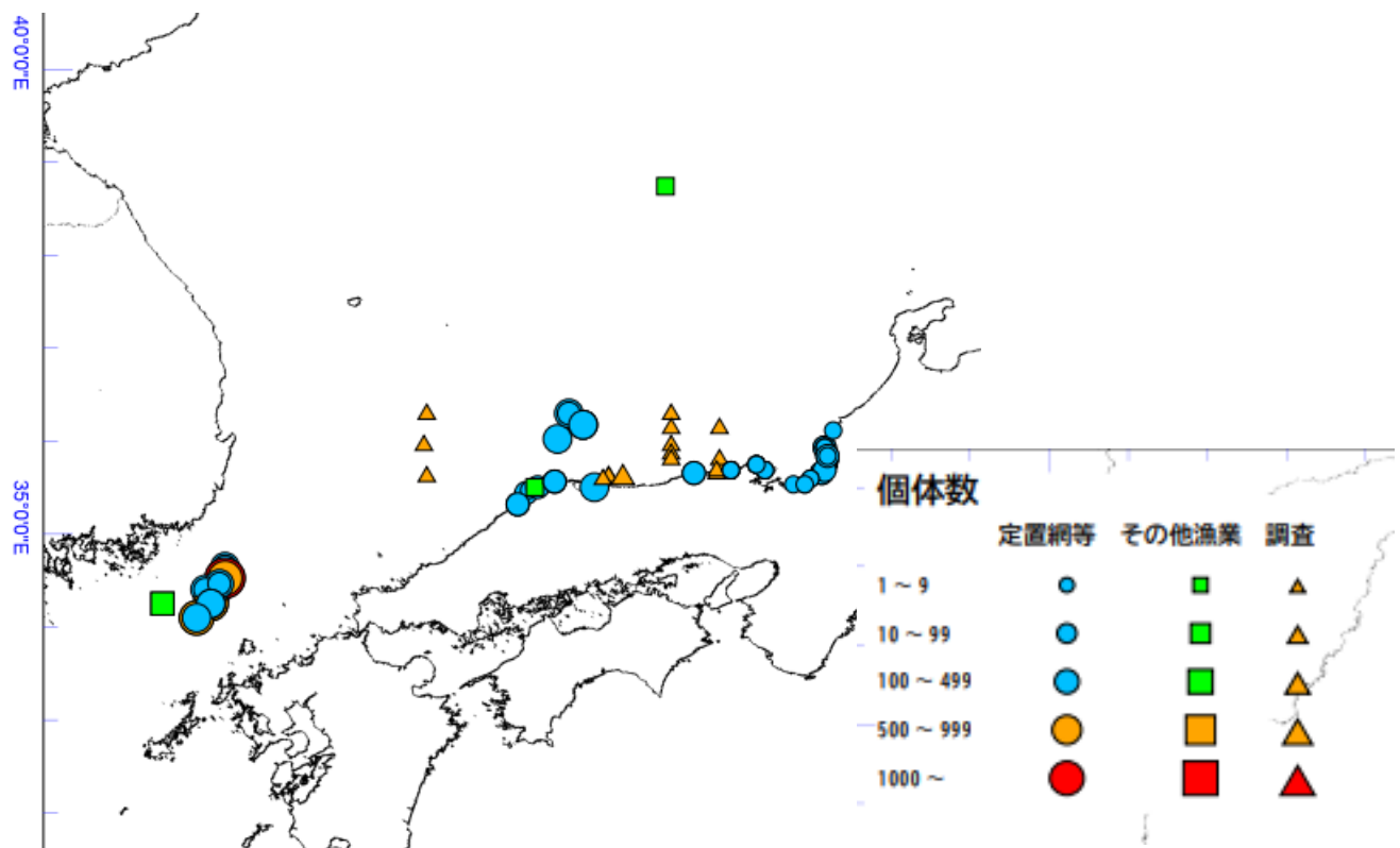
図 大型クラゲ出現分布（JAFIC 資料より抜粋）
