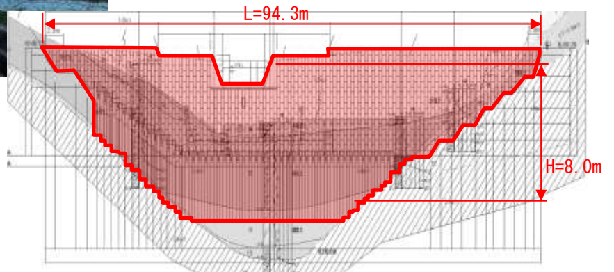
砂防堰堤（正面図）
