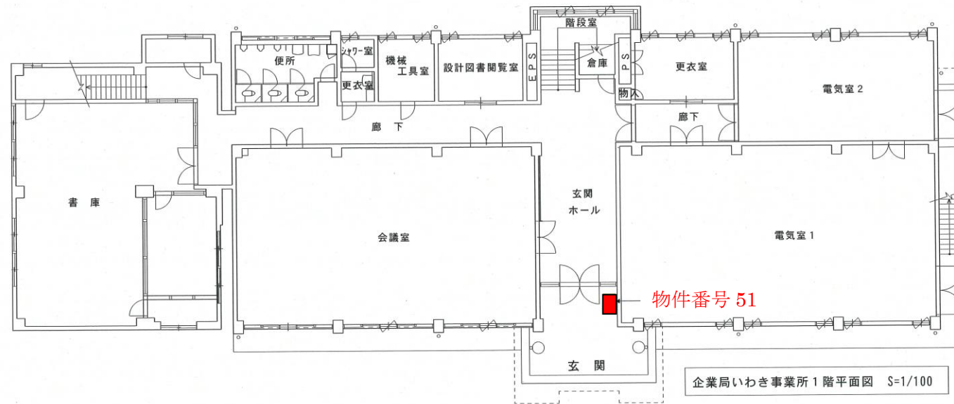
企業局いわき事業所庁舎配置図
