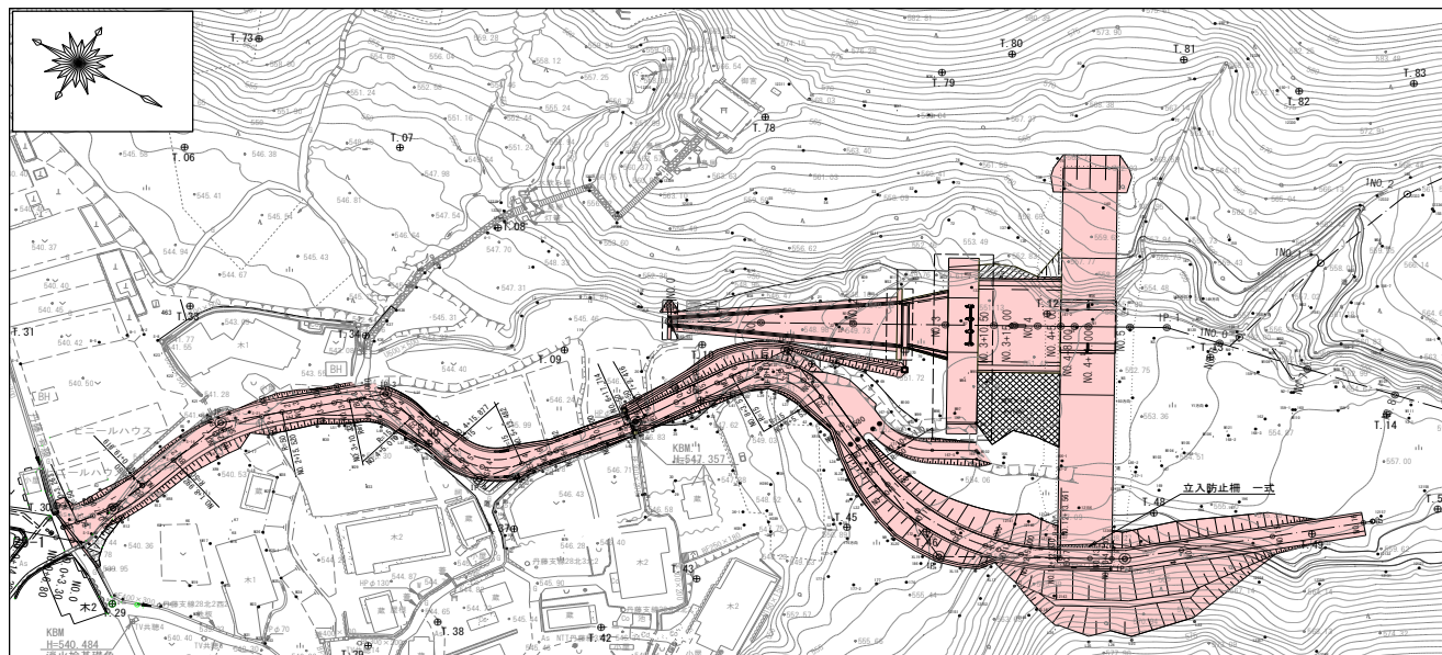
▲ 平面図
