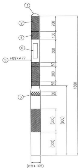
参考図 S=1/10
