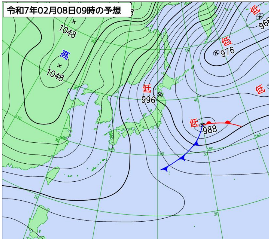
予想天気図
