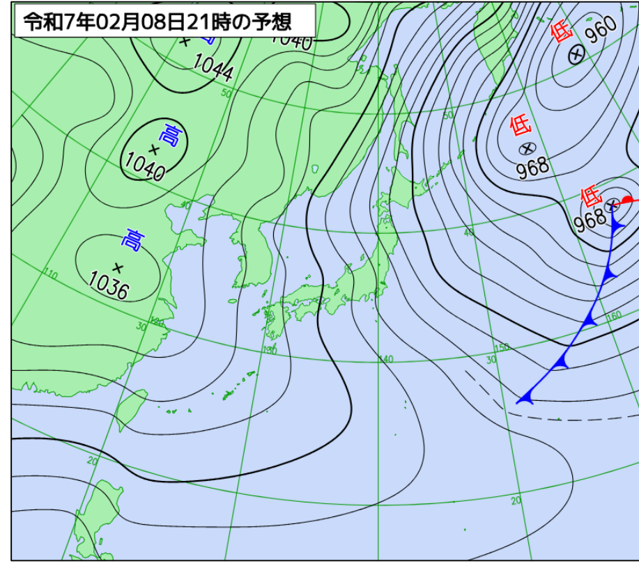
予想天気図
