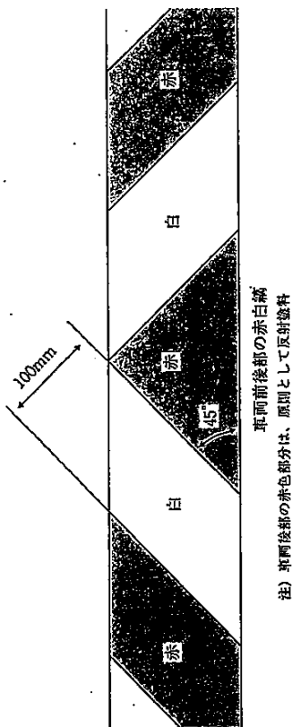
図一1 道路維持作業用自動車の塗色要領図
