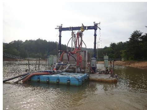
ため池の底質をポンプ浚渫する状況
