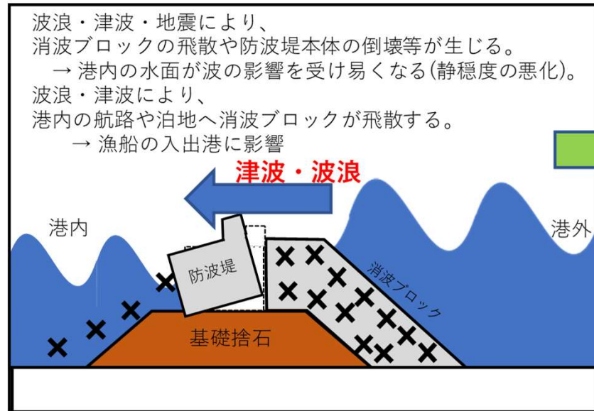
防波堤断面
