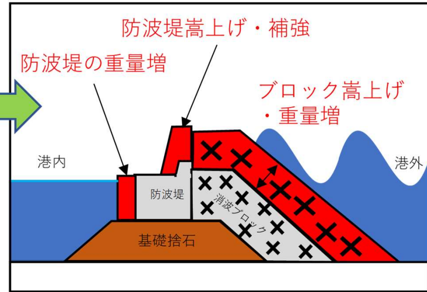
防波堤断面
