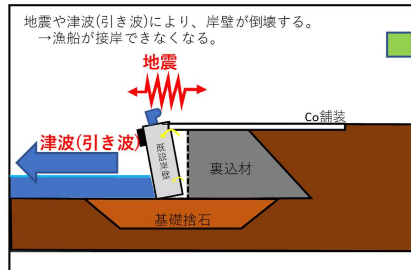
岸壁断面
