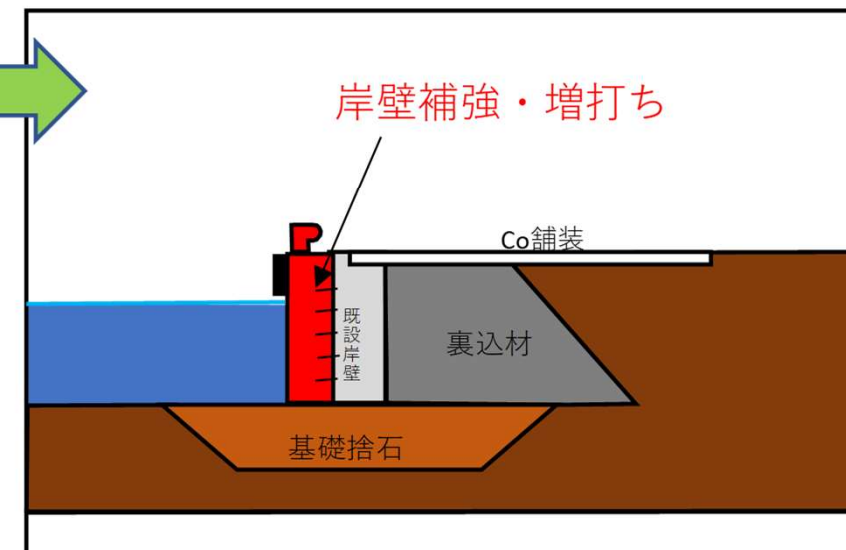
岸壁断面
