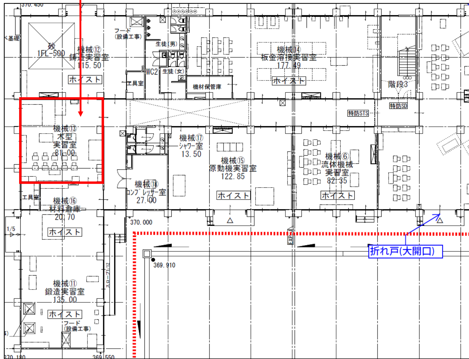
福島県立白河実業高等学校 新実習棟平面図
