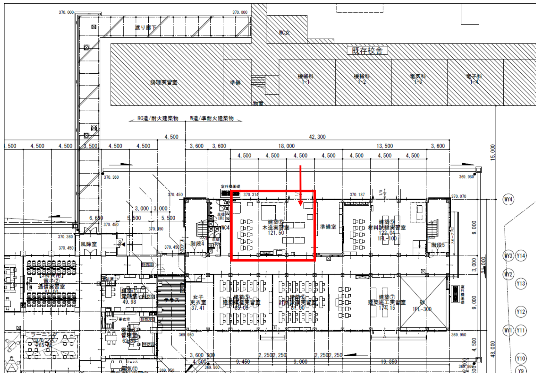
福島県立白河実業高等学校 実習棟平面図
