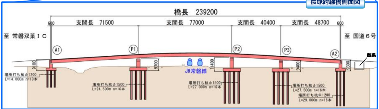
長塚跨線橋側面図
