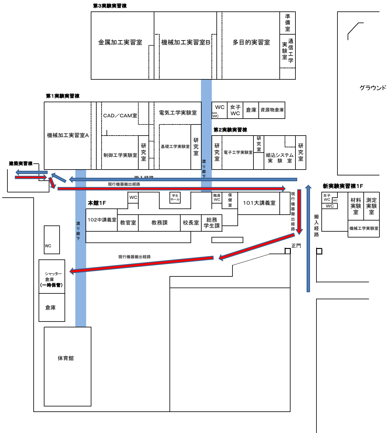
テクノアカデミー郡山 手押しかな盤搬入搬出経路図
