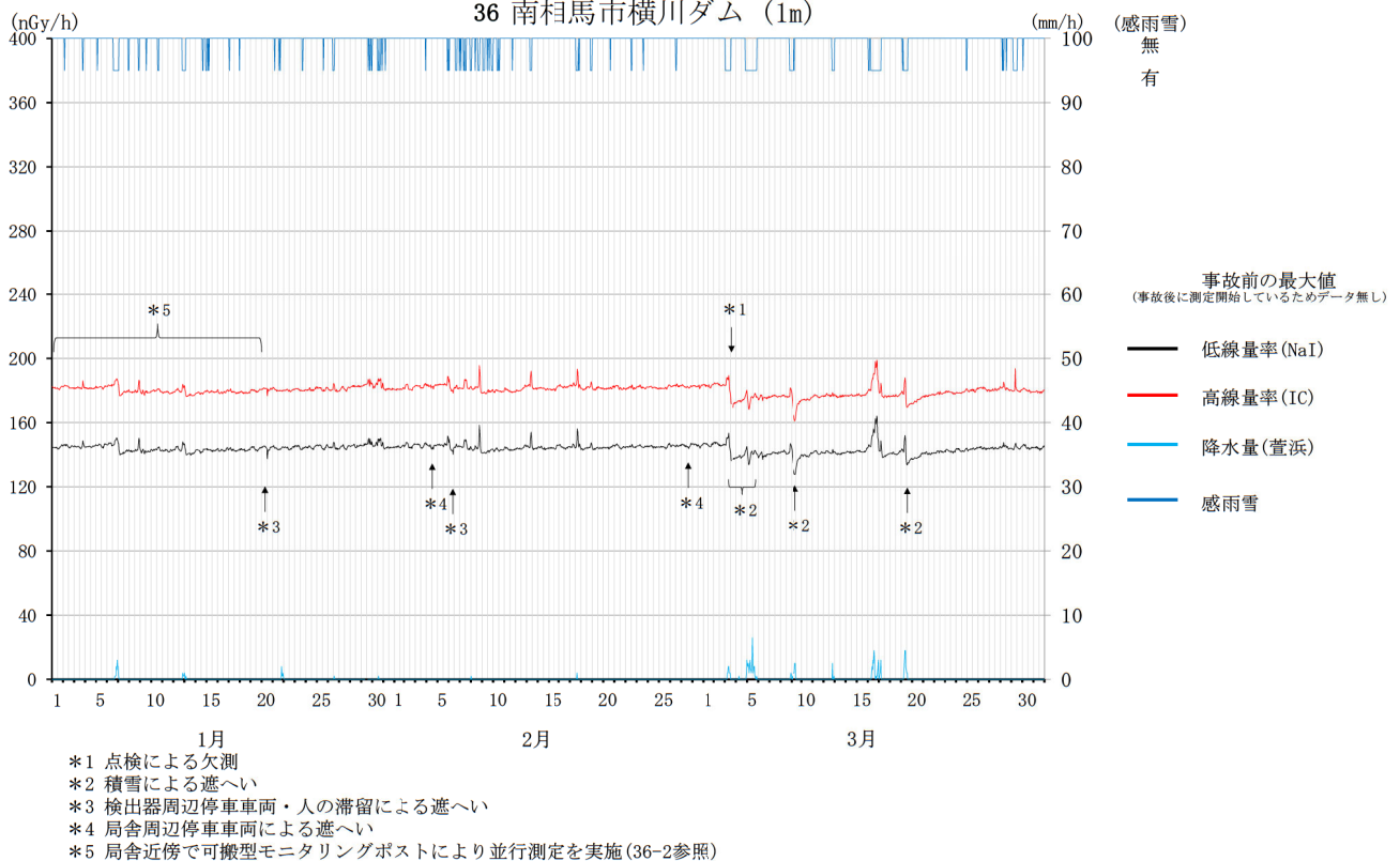
空間線量率の変動グラフ 36 南相馬市横川ダム (1m)
