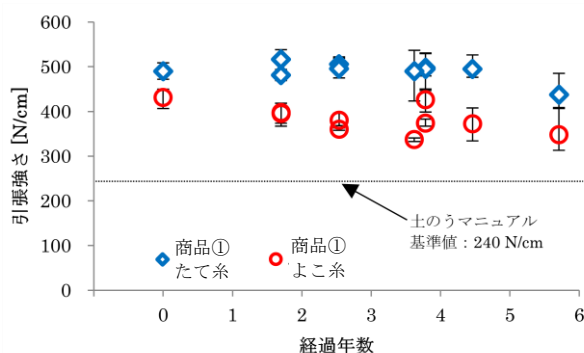
図5-17 遮光保管された除去土壌等保管容器(耐候性大型土のう) 本体生地引張試験の結果
