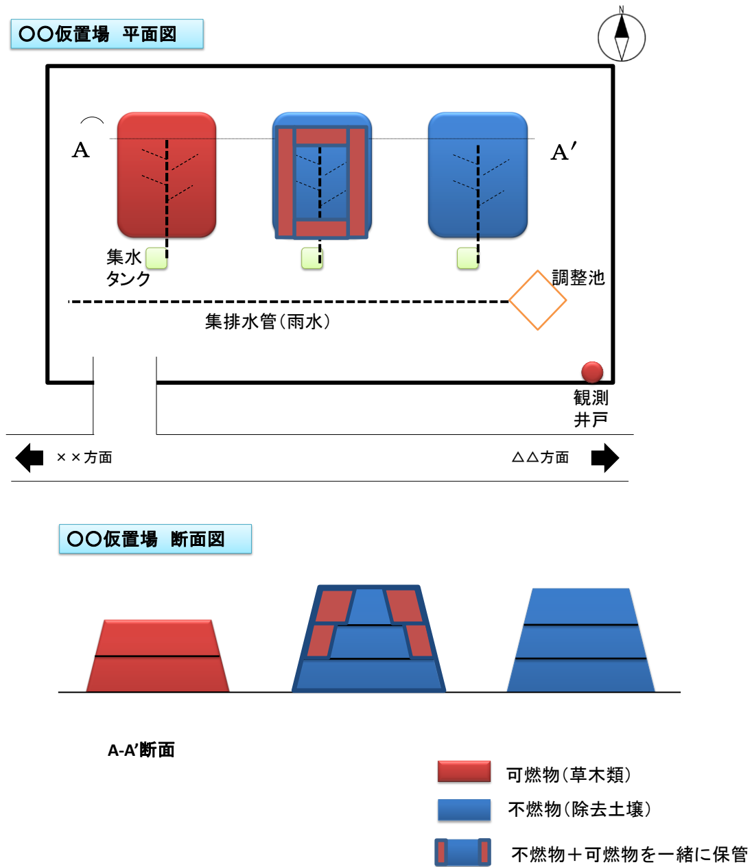
図 2-31 平面図、断面図の例
