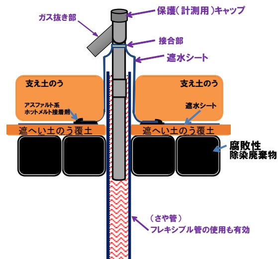
図 2-26 ガス抜き管変形・転倒軽減構造の採用例
