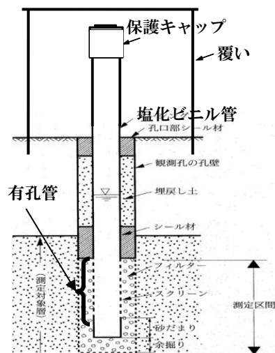
図 2-28 地下水観測孔の例
