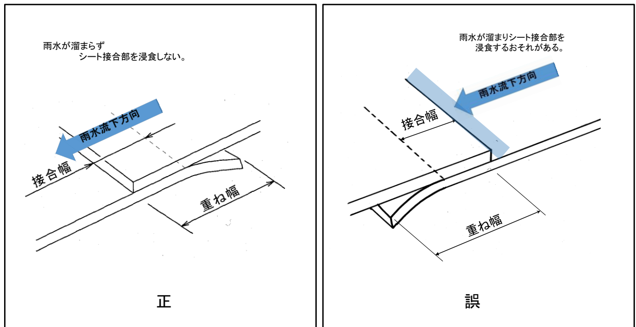
図 2-15 シート接合部の重ね合わせ方向
