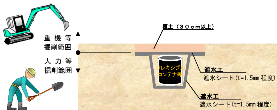
図 5-5 現場保管における積み準備の施工例
