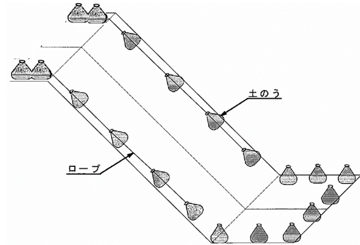
図 2-20 重し土のうによる養生例
