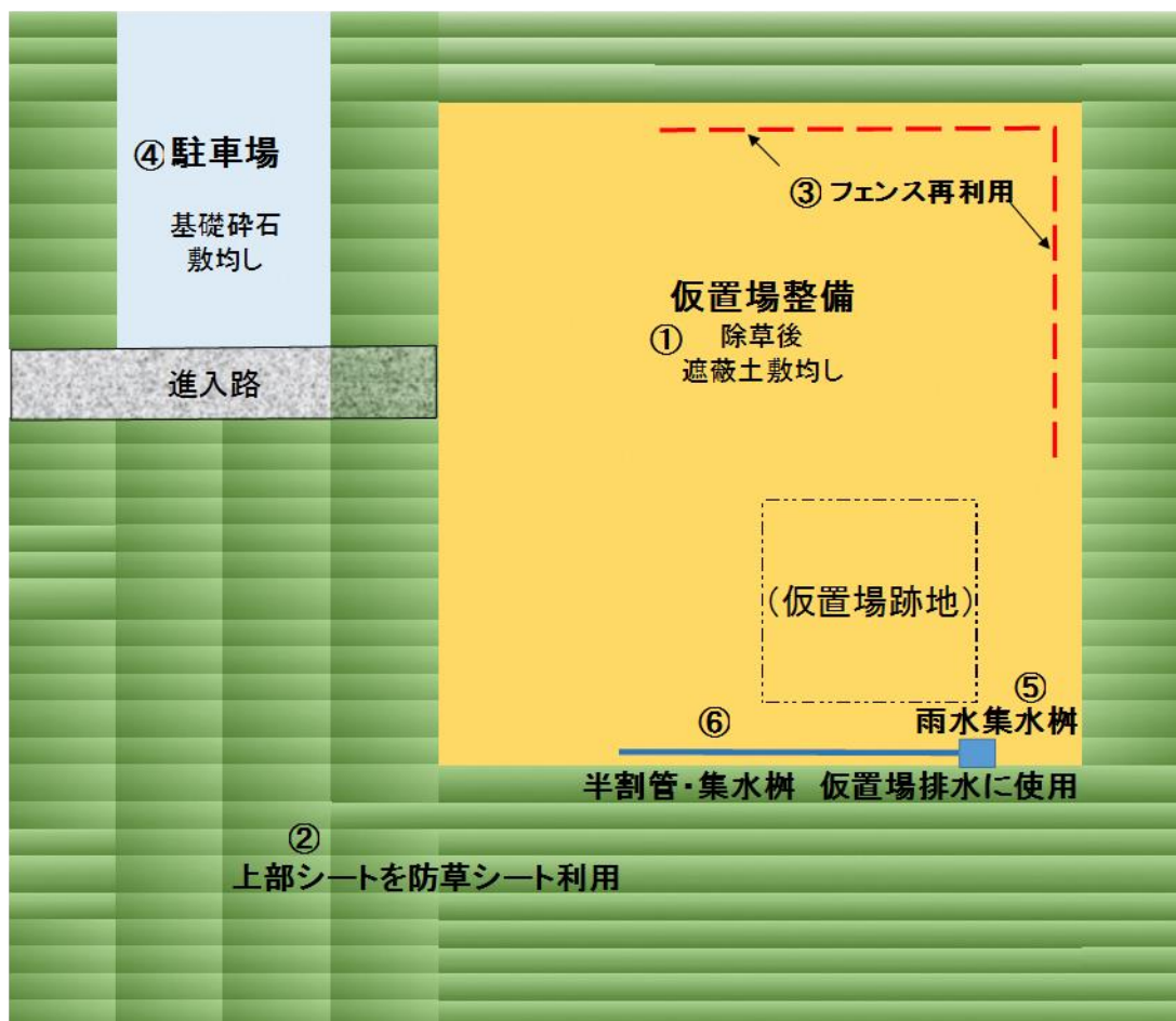
図 6-2 仮置場平面概要図
