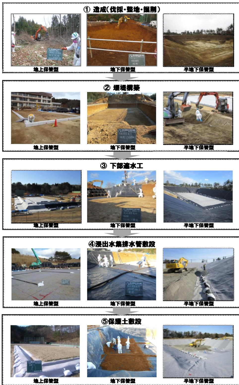
図 2-2 仮置場の施工の流れ ―モデル実証事業の例― (福島第一原子力発電所事故に係る避難区域等における除染実証業務 報告書 (独立行政法人 日本原子力研究開発機構 平成 24 年 6 月) より引用)
