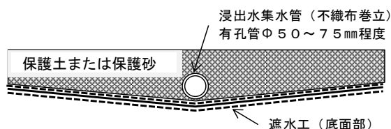
図 2-22 浸出水集水管の例
