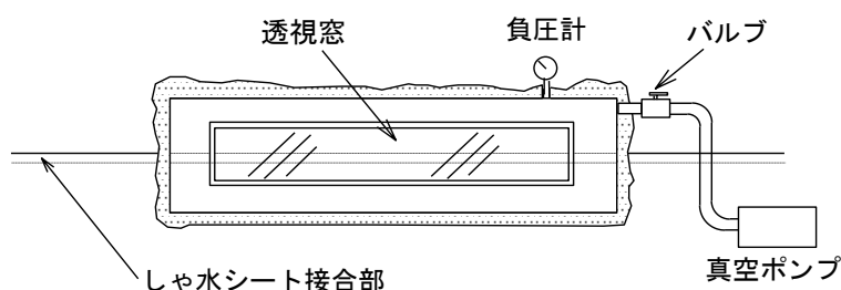
図 2-18 気密式検査 減圧式（バキューム法）の例
