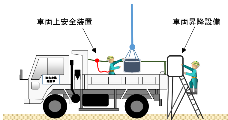
図 5-22 積込み時安全対策（車両上安全帯、車両昇降設備）事例
