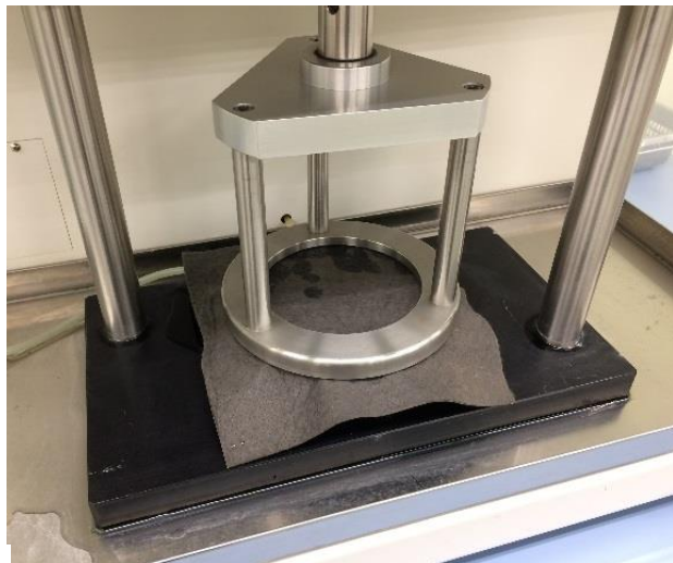
図 5-21 通気性防水シートの耐水圧試験
