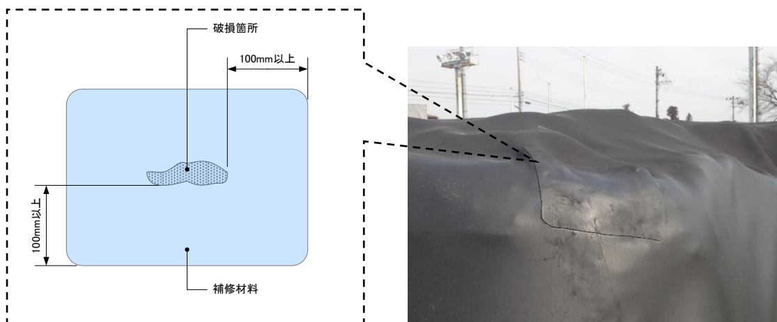
図 3-5 上面部の遮水シートを補修した例
