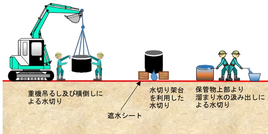
図 5-12 保管容器の水切り施工例
