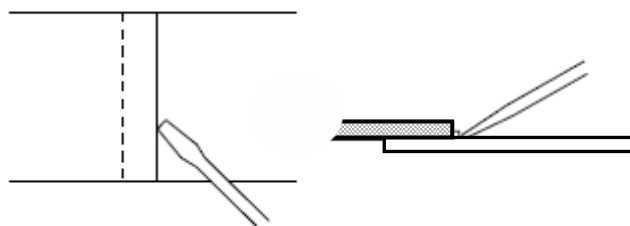
図 2-16 検査棒挿入検査（ドライバークHECK）の例
