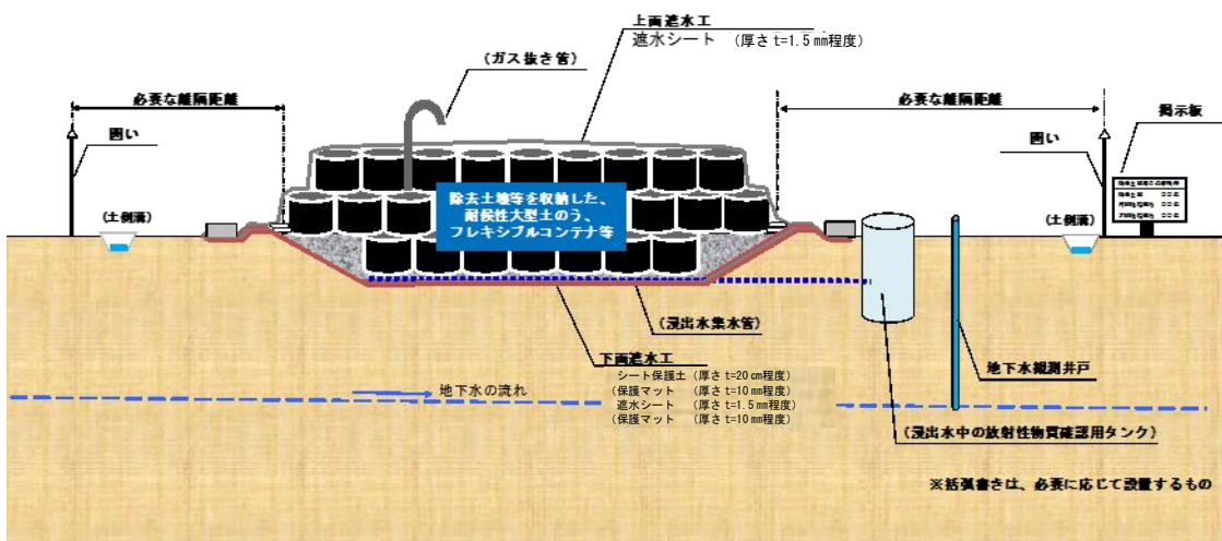
図 2-1 仮置場の標準断面構造の例
