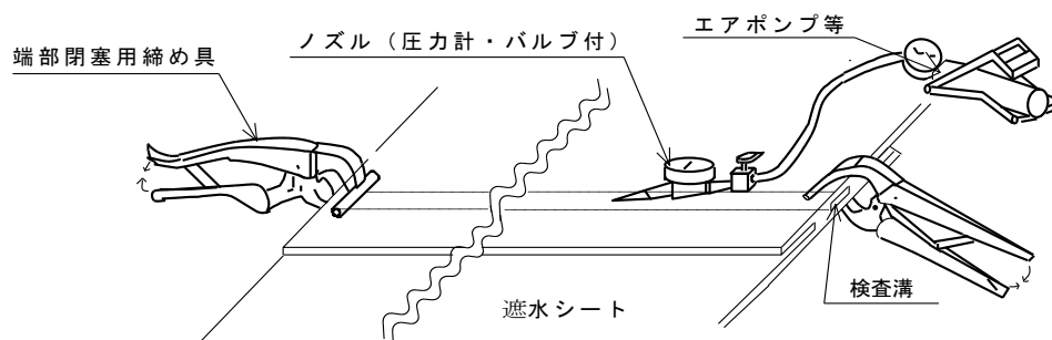
図 2-17 気密式検査 加圧式（ダブルシーム法）の例
