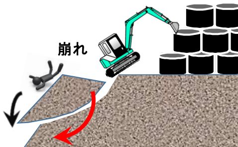
図 5-6 地上型の場合の事故例(1)
