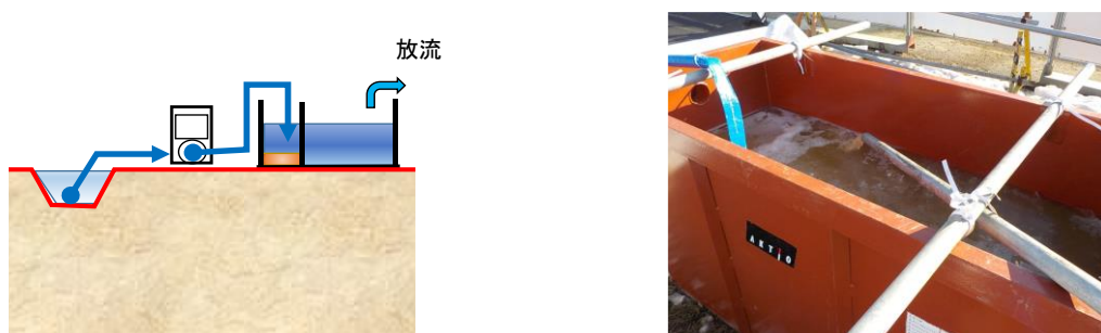
図 5-14 排水処理施工例
