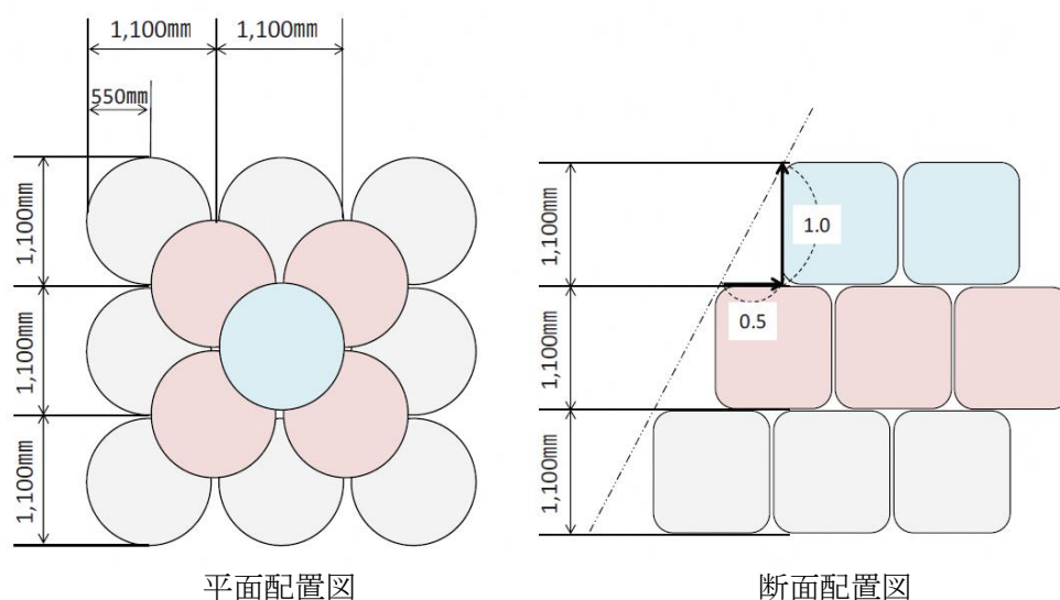
図 2-12 容器の積み上げ配置図（容器の例）
