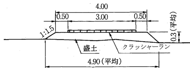
図 2-32 工事用仮設道路標準断面図の例
