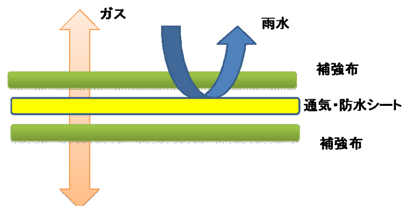
図 2-19 通気性防水シート構造図
