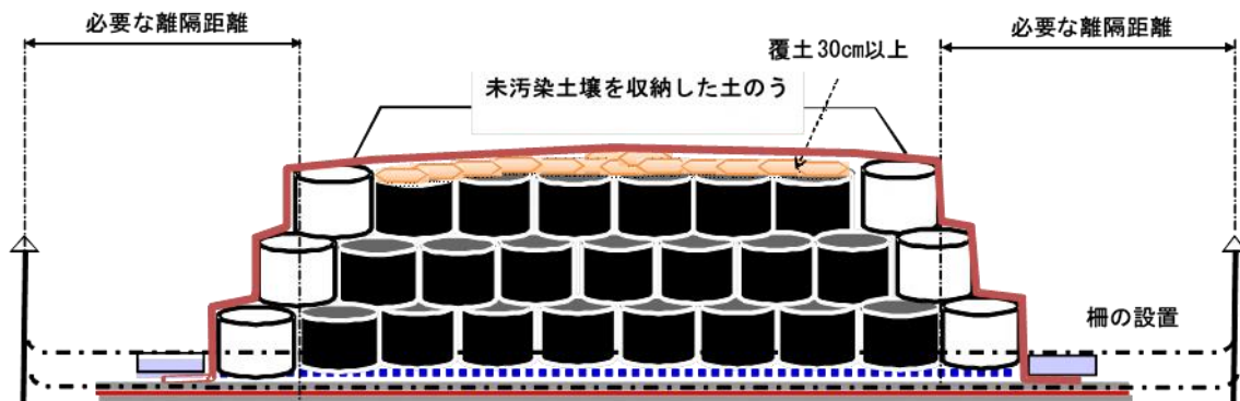
図 2-3 遮へいを実施する場合の例
