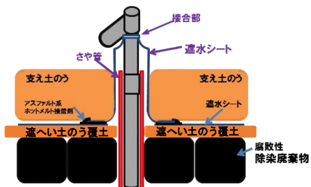
ガス抜き管接合部の雨水対策（概略構造図）
