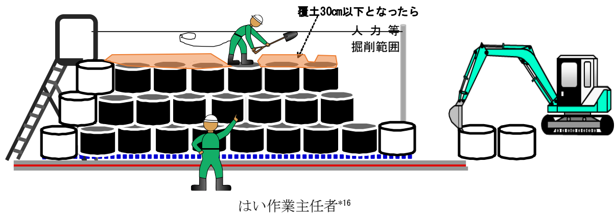
図 5-4 仮置場における積み準備の施工例
