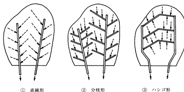
図 2-23 集排水管の配置例
