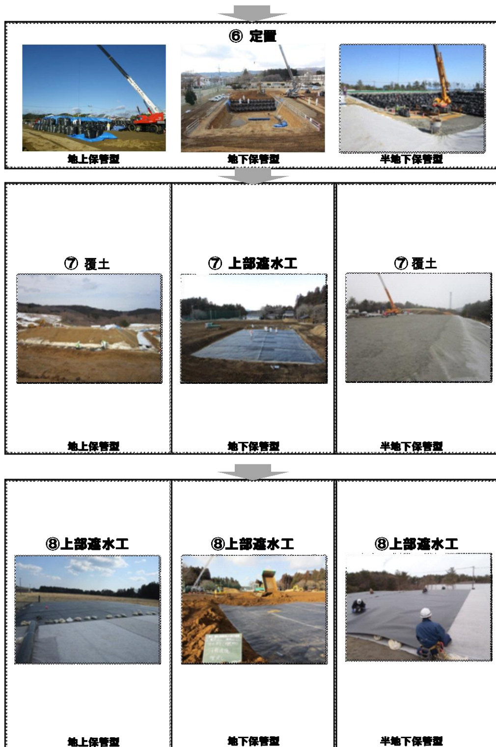
図 2-2 仮置場の施工の流れ ―モデル実証事業の例― (続き)
