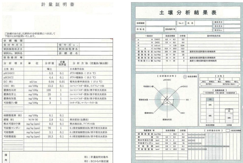
図 6-6 土壌分析結果例
