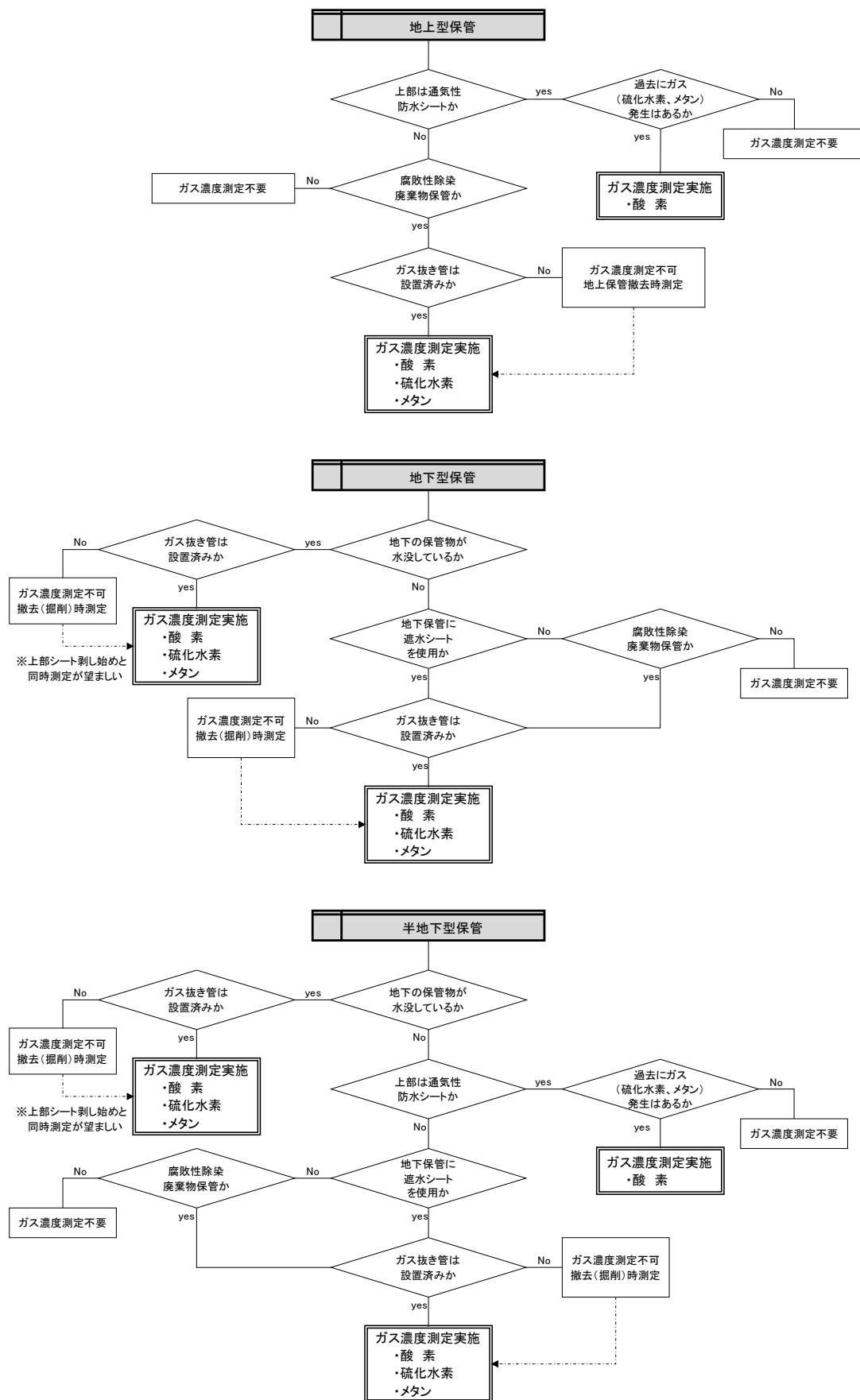
図 5-1 ガス測定区分のフローチャート
