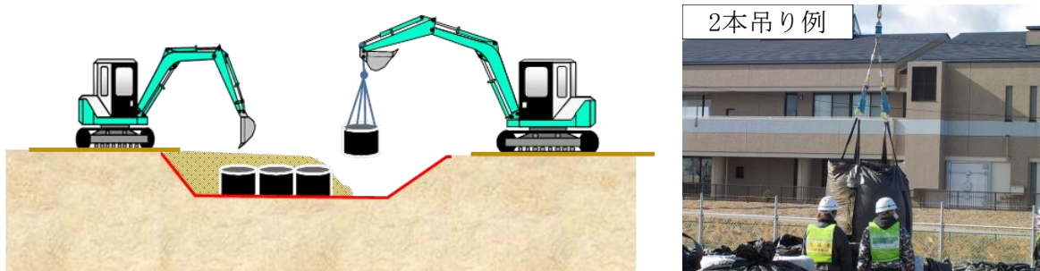
図 5-11 保管容器掘り起こし例
