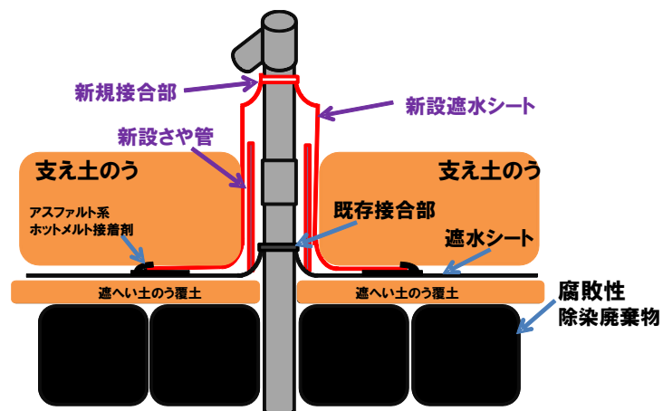
図 3-7 ガス抜き管接合部の雨水対策（補修例）
