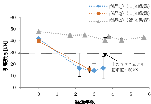
図5-19 遮へい用土のう(耐候性大型土のう) 吊ベルト引張試験の結果
