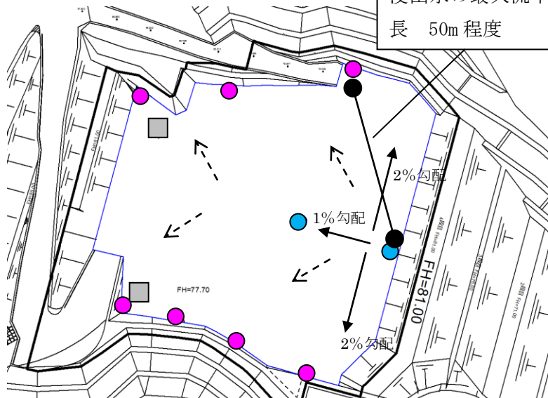
図 2-21 (1) 堅管、法面ガス抜き管の平面配置
