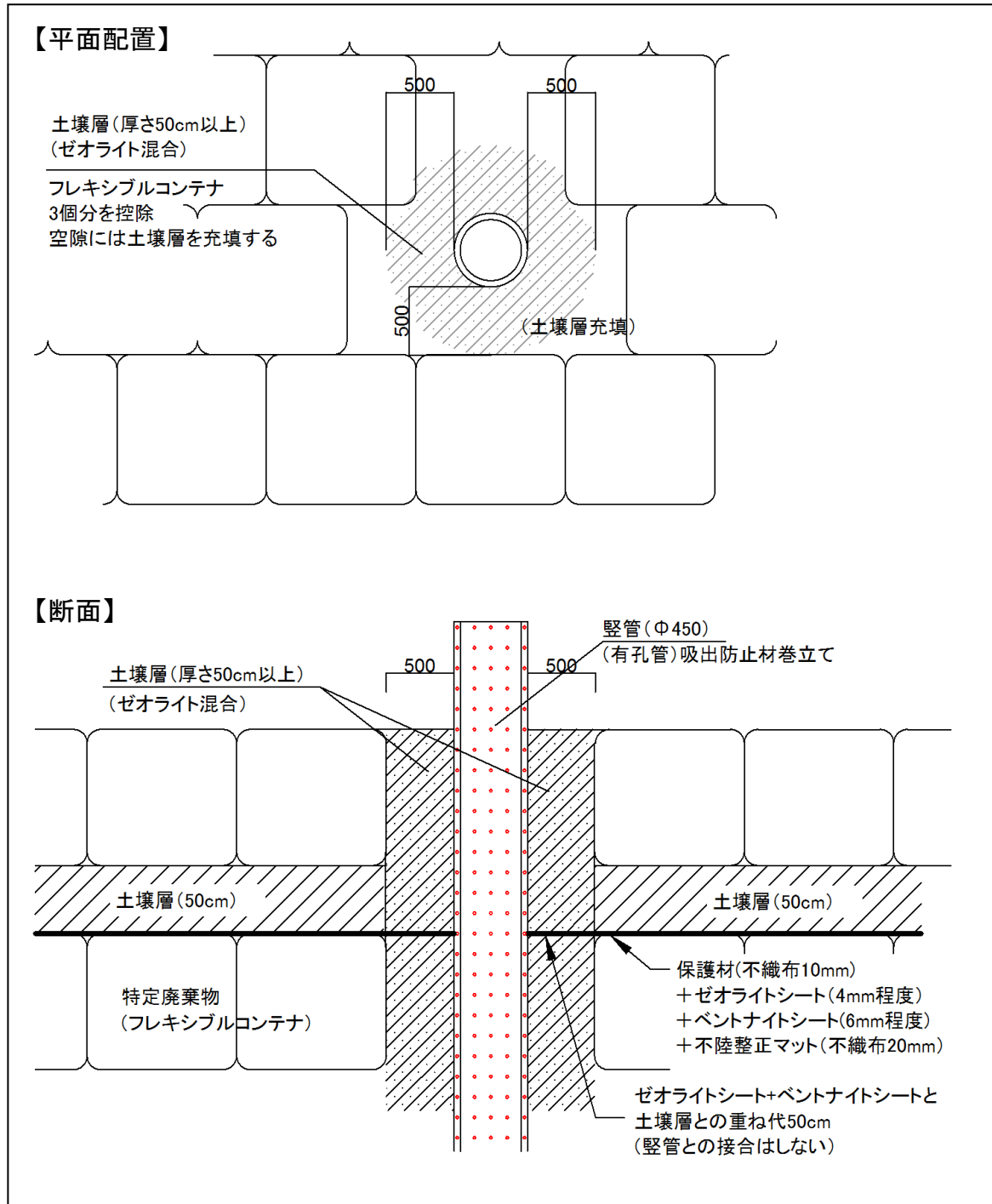
図 2-22 堅管の標準構造
