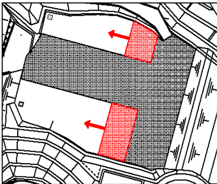
図 2-17 排水勾配の上流側からの埋立順序 (例)
