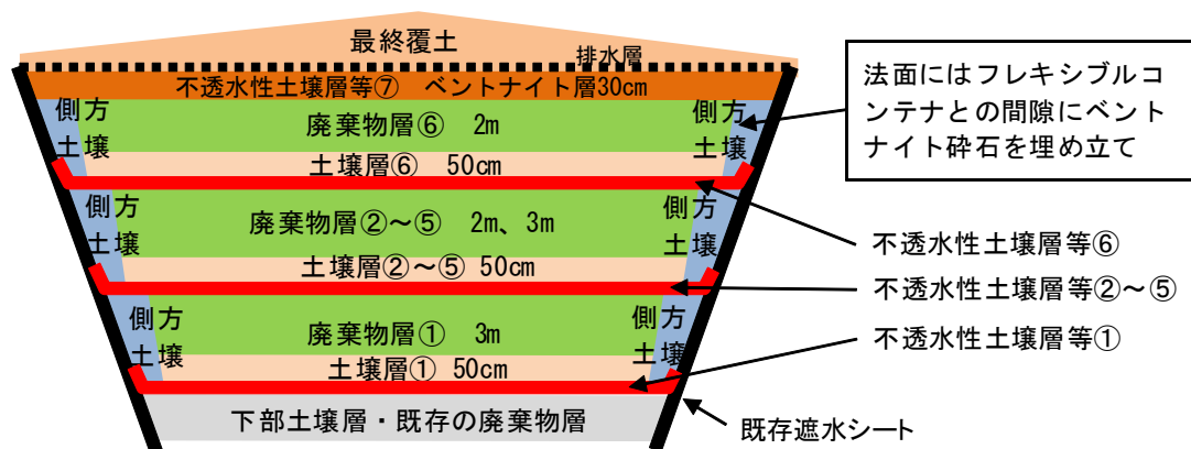
図 2-11 セメント固型化した廃棄物の埋立層
