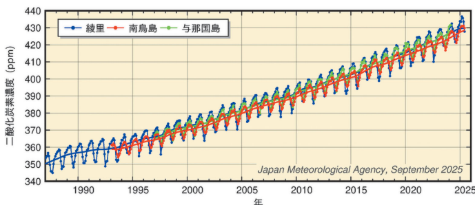
出典：気象庁ホームページ 「大気中二酸化炭素濃度の経年変化」
