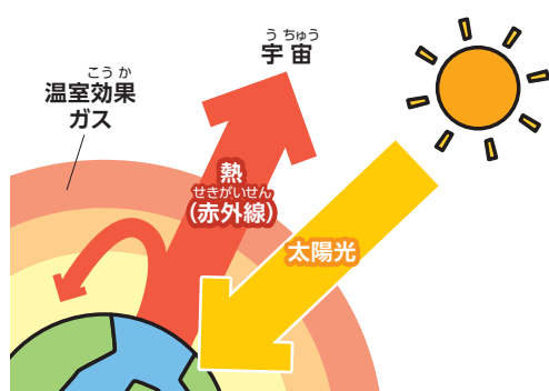
〈バランスのとれた大気の状態〉
