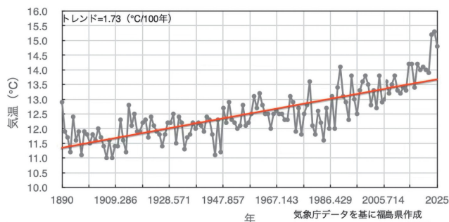
福島の年平均気温
