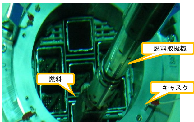
(写真 16) キャスクからの燃料取り出し作業
