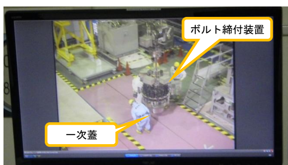
(写真5) 一次蓋とボルト締付装置（遠隔操作室モニタを撮影）
