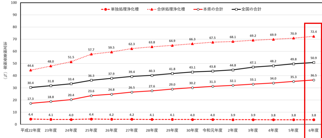
図7 浄化槽の法定検査受検率の推移
