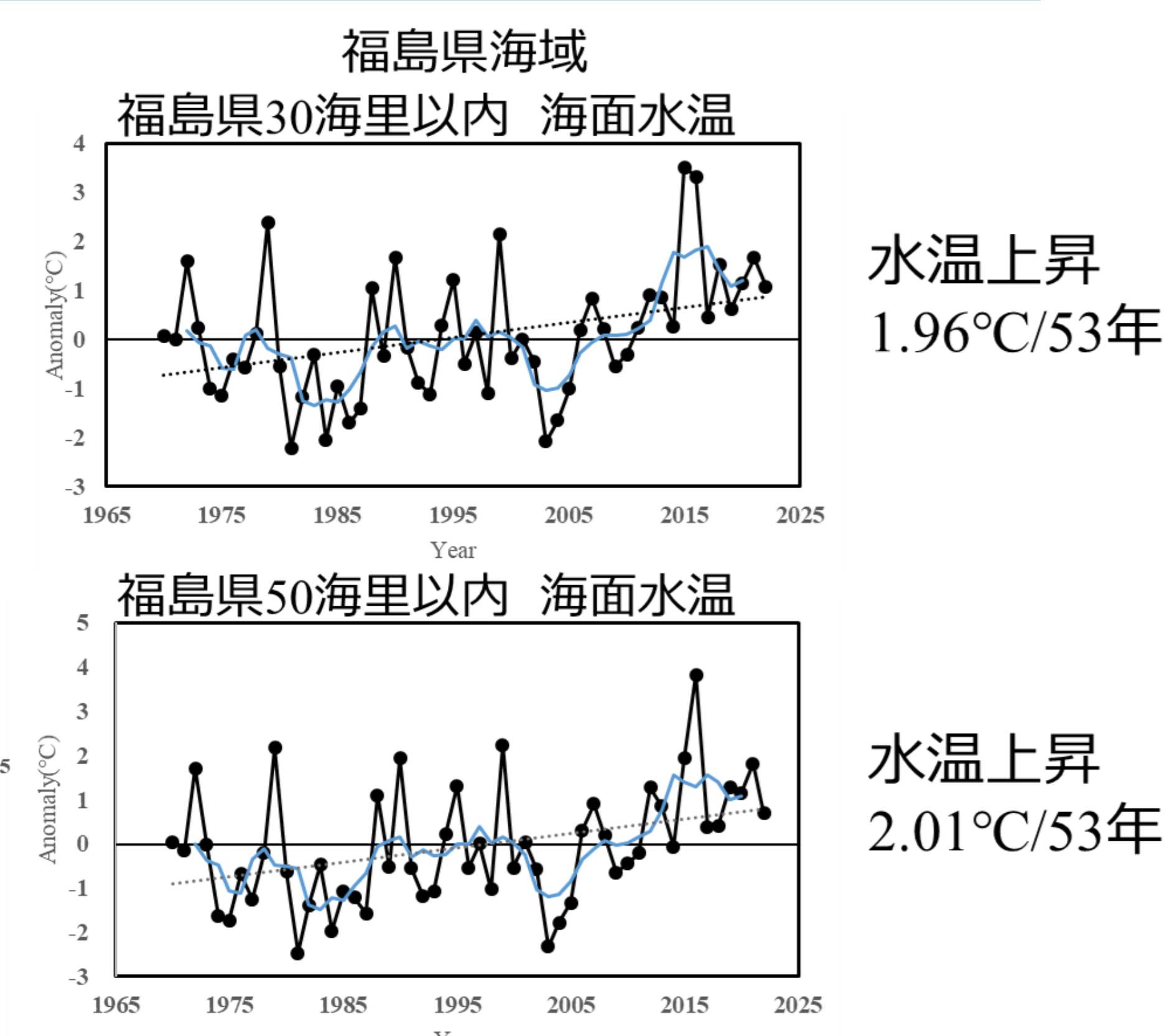
図5 気象庁データと福島県海洋観測データを用いた海面水温の長期的な変動傾向の比較(1970~2022年,参考となる成果より抜粋)
