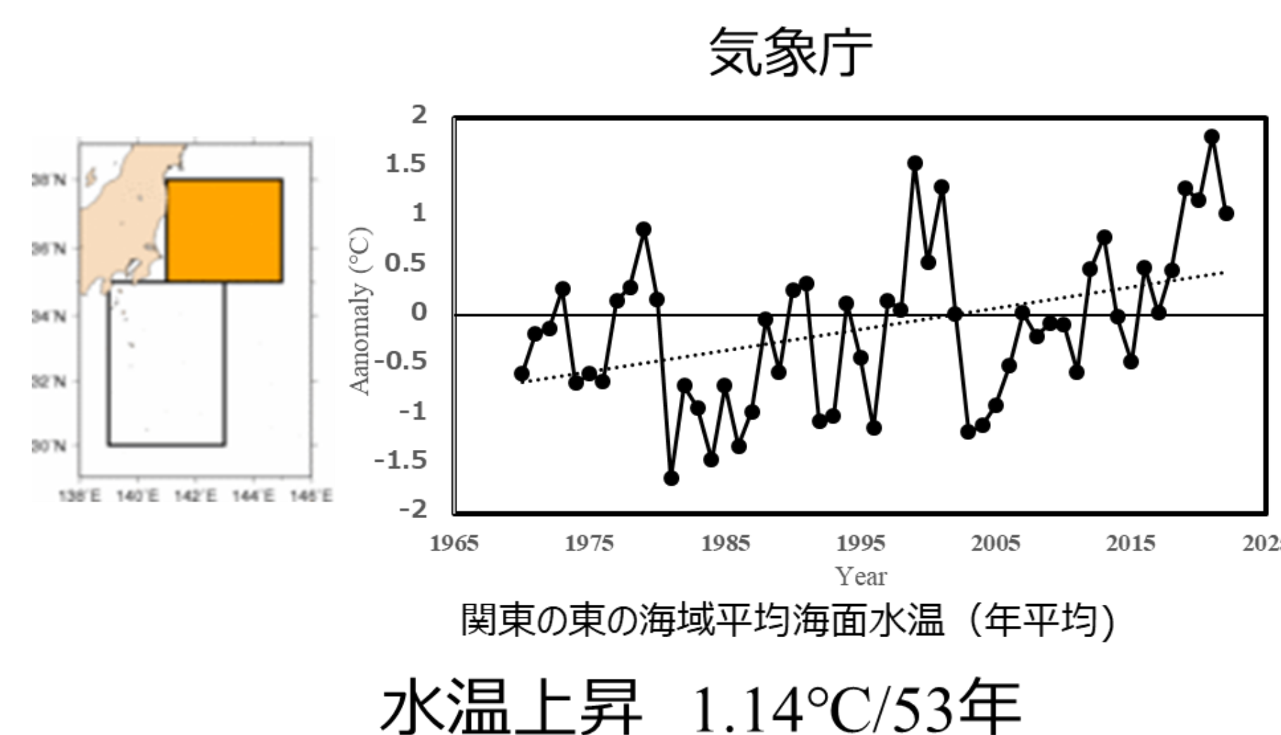
図5 気象庁データと福島県海洋観測データを用いた海面水温の長期的な変動傾向の比較(1970~2022年,参考となる成果より抜粋)
