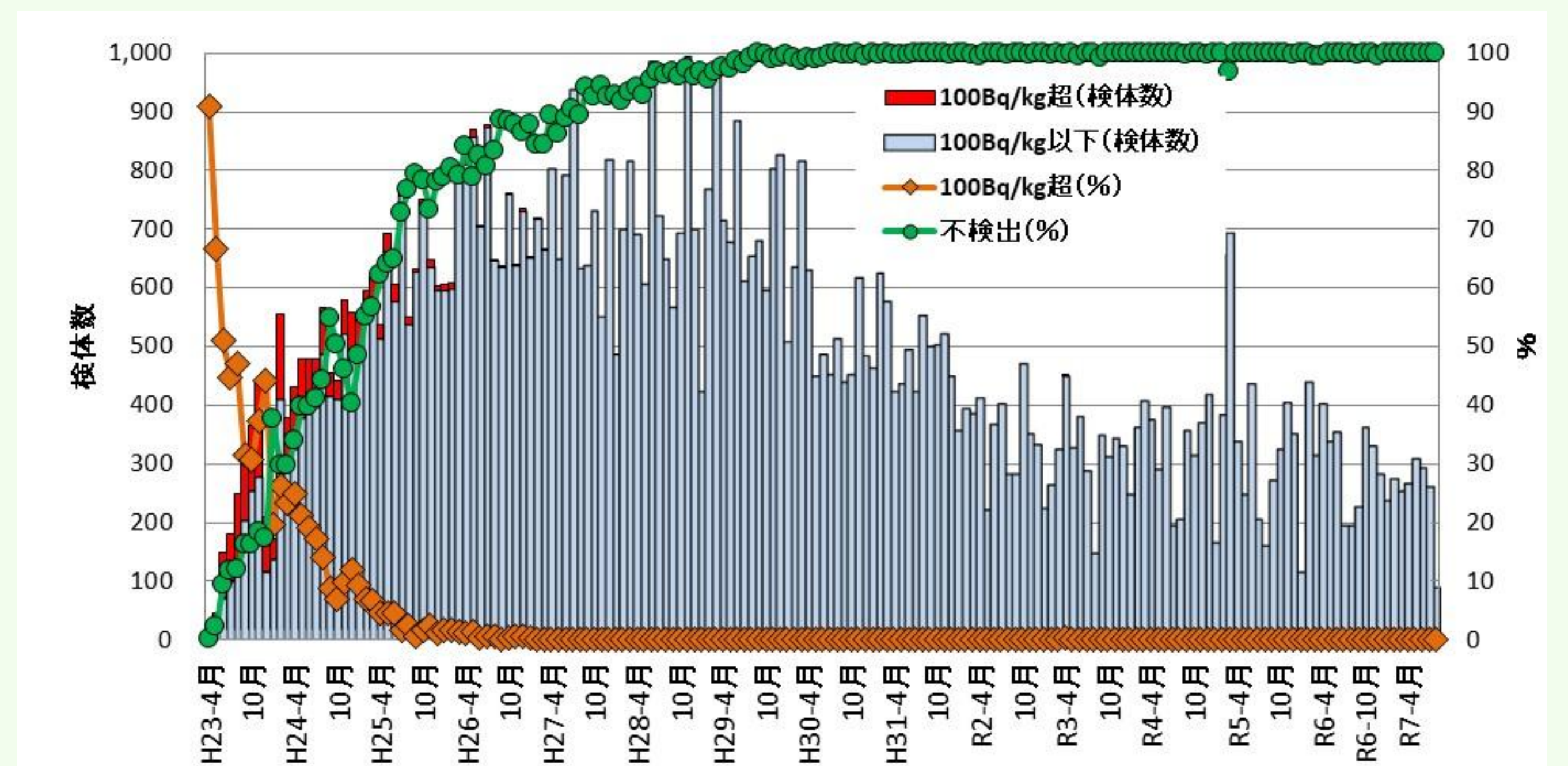
図3 月別の検体数及び検体数の割合(100Bq/kg超、不検出)の推移
