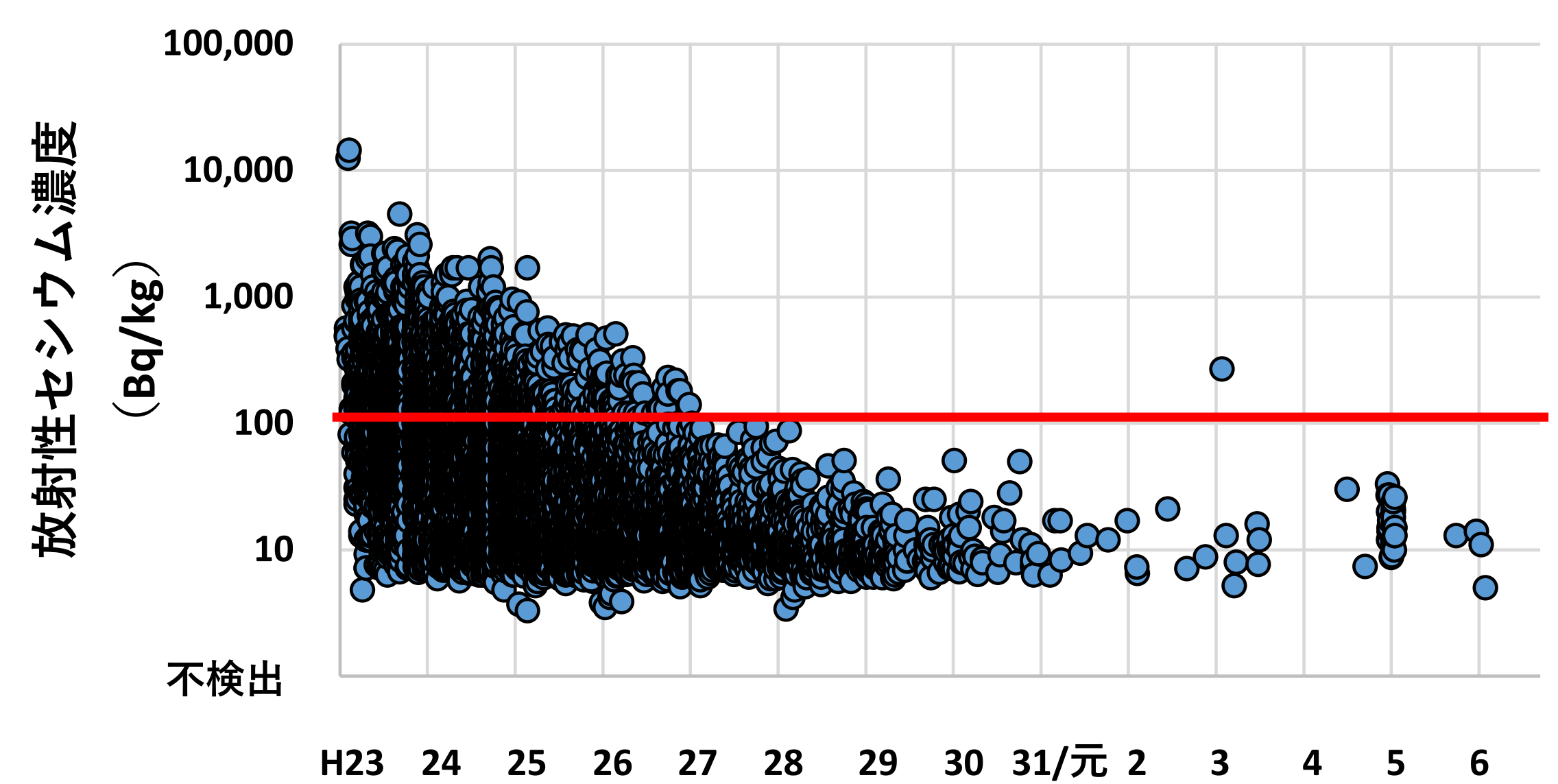
図2 魚介類の放射性セシウム濃度の推移
