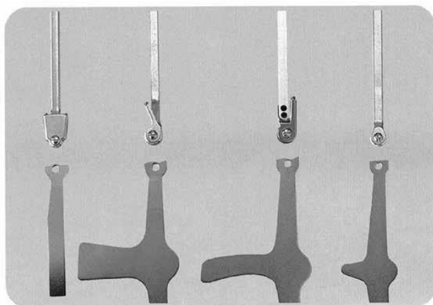
↑ダブルクレンザック ↑クレンザック
