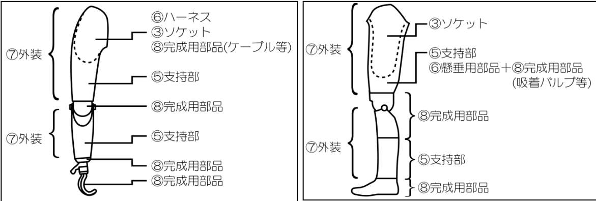
↑ 殻構造上腕義手の構成例
