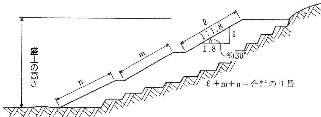
図 1(10)-1 盛土の高さ
