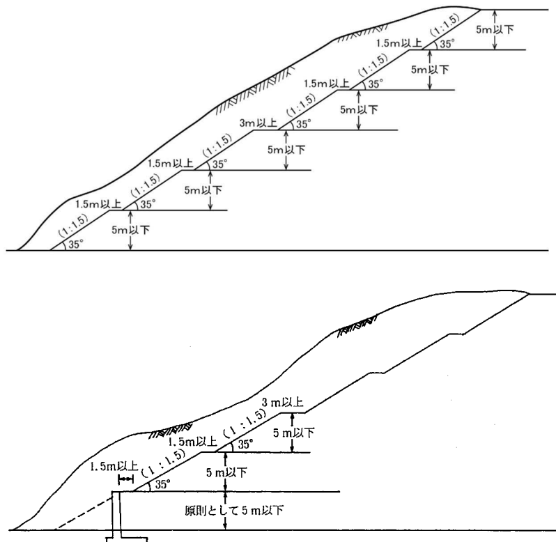
図 1(7)-2 長大法（切土）の参考断面図（法尻に鉄筋コンクリート擁壁を設置する場合）
