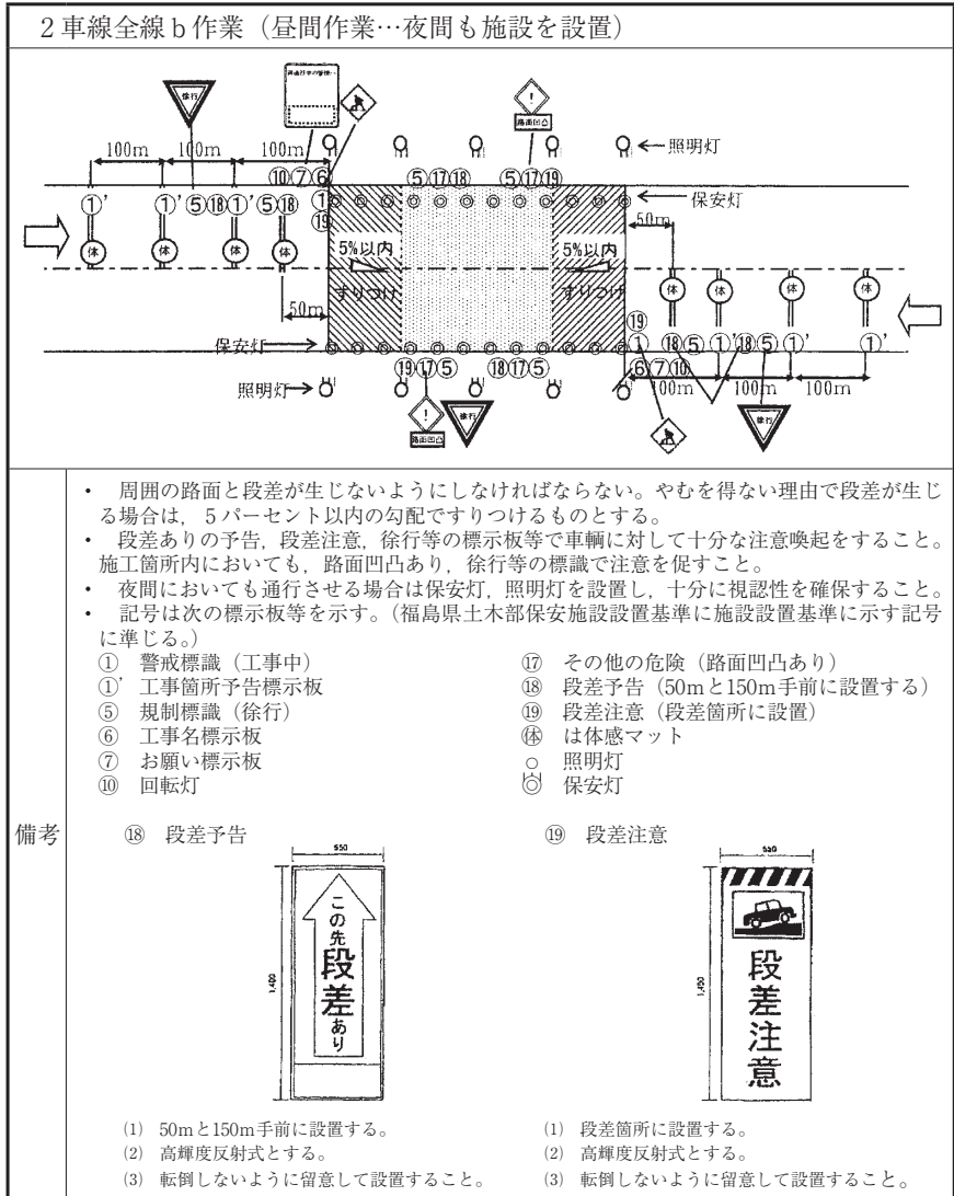
保安施設設置図
