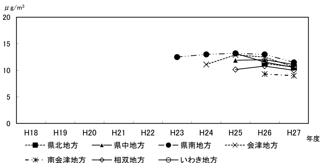
図-11 微小粒子状物質(年平均値)の経年変化
