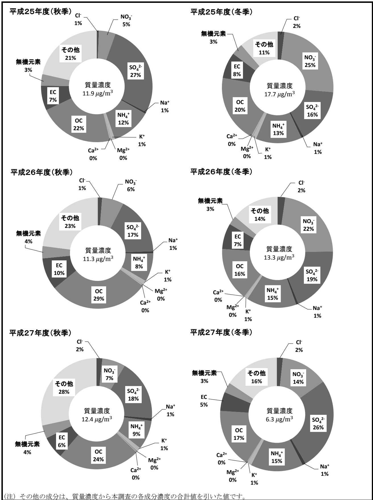
図-17 会津若松局におけるPM2.5成分組成の経年変化
