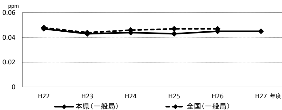
図-4 光化学オキシダント濃度の推移
